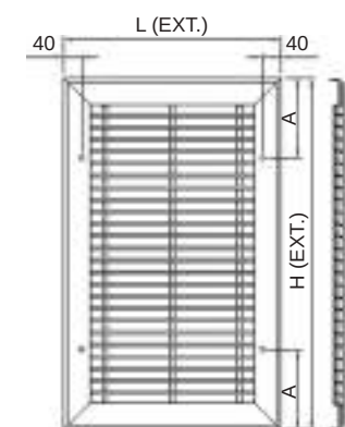
RPK REJILLA FIJA Y TORNILLOS VISTOS
