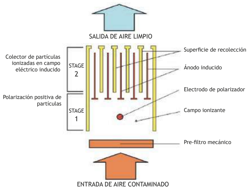
Principio operativo del filtro electrónico Crystall Sabiana IFEMEC
