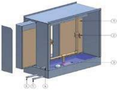
Módulo Adiabático TECNAVENT MA
